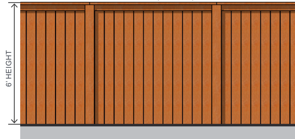
REAR ELEVATION (N.T.S.) - TO FACE LOT
